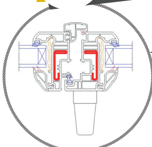
Poignée décentrée Sans battement
